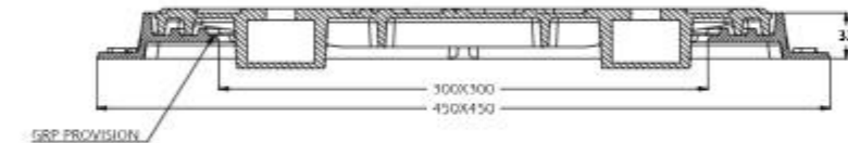
SECTION A-A
